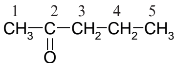
2-пентанон
