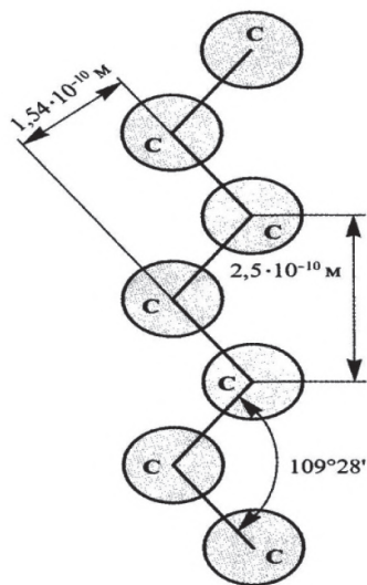
Расми 5. Шакли занҷири ҳептан.
