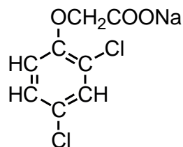
2,4-дихлорфеноксиатсетати натрий
