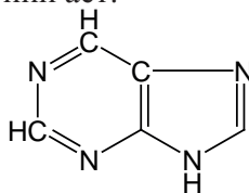
пурин
