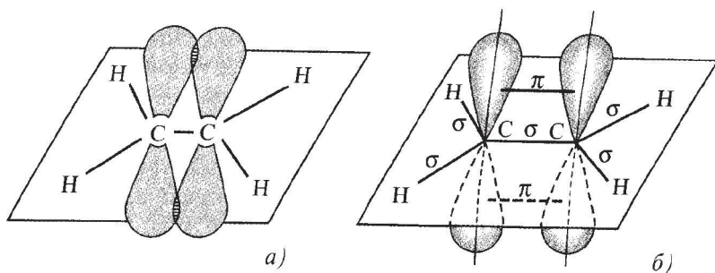
Расми 9. Схекаи пайдоиши π-банд дар молекулаи этилен
