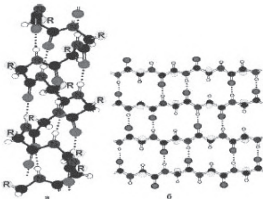
Расми 34. Конфигуратсияи занҷирҳои полипептиди: а) \alpha -спирал, б) \beta -структура
