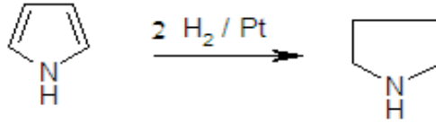
пиррол
