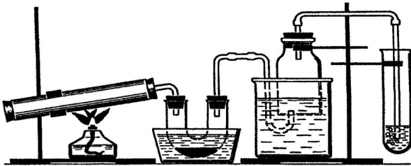
Расми 23. Тафсонии ангиштсанг дар муҳити беҳаво
