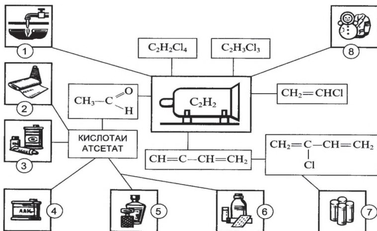
Расми 15. Истифодабарии ацетилен ва пайвастиҳои он: 1-барои кафишер ва буридани металҳо; 2-ҳосил кардани нахи сунъӣ; 3-рангубор; 4-лакҳо; 5-атр ва моддаҳои атторӣ; 6-дорувор; 7-каучуи хлорпренӣ; 8-поливинилхлорид.
