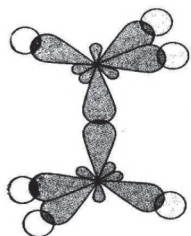
Расми 2. Ҳосилшавии молекулаи этан дар натиҷаи пӯшидашавии ду абри электронии хибридуи атомҳои карбон
