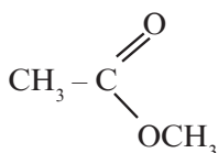
эфири мураккаби метилатсетат
