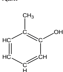
орто-крезол
