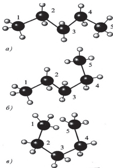
Расми 6. Моделҳои куррагию меҳвари молекулаи пентан.
