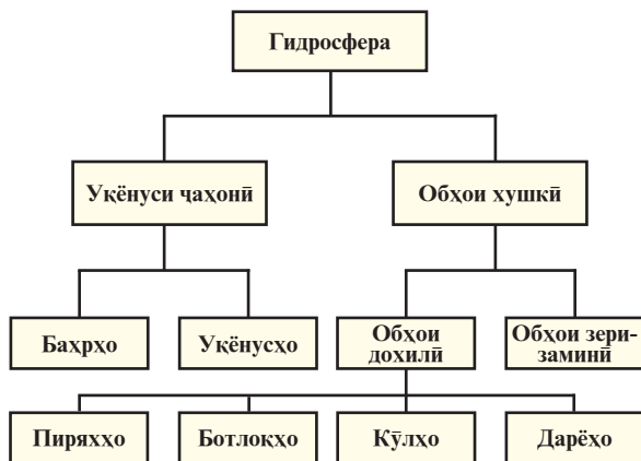
Таркиби гидросфера
