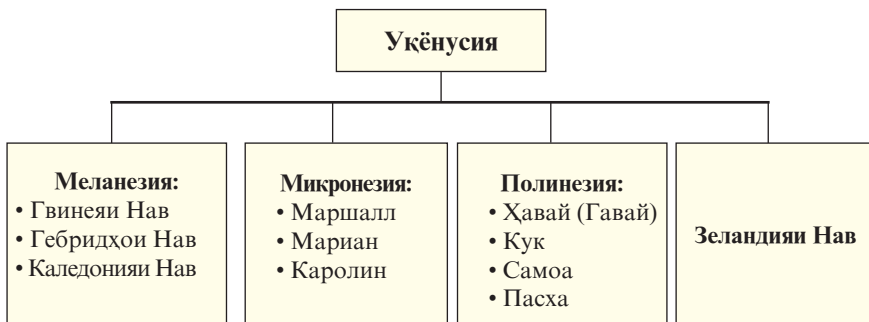
Таркиби Укёнусия
