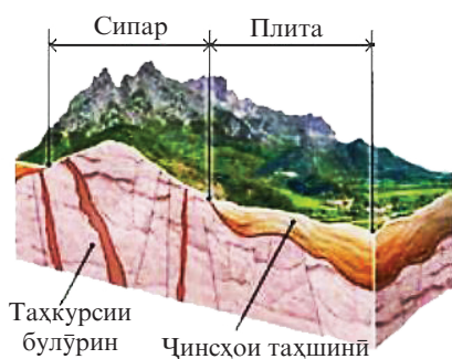
Соҳти платформаҳо
